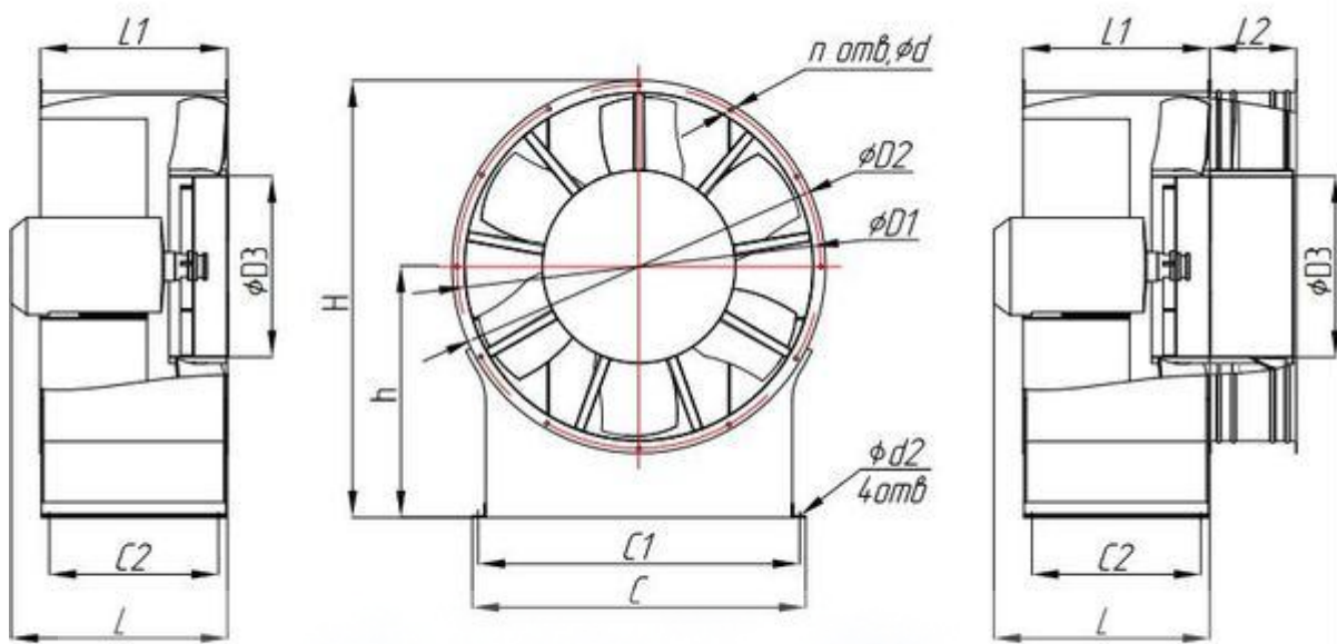
Габаритные и присоединительные размеры вентиляторов ВО 25-188-6,3 12,5
