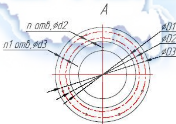
Габаритные и присоединительные размеры вентиляторов крышных типа ВКРФ 3.55-12.5
